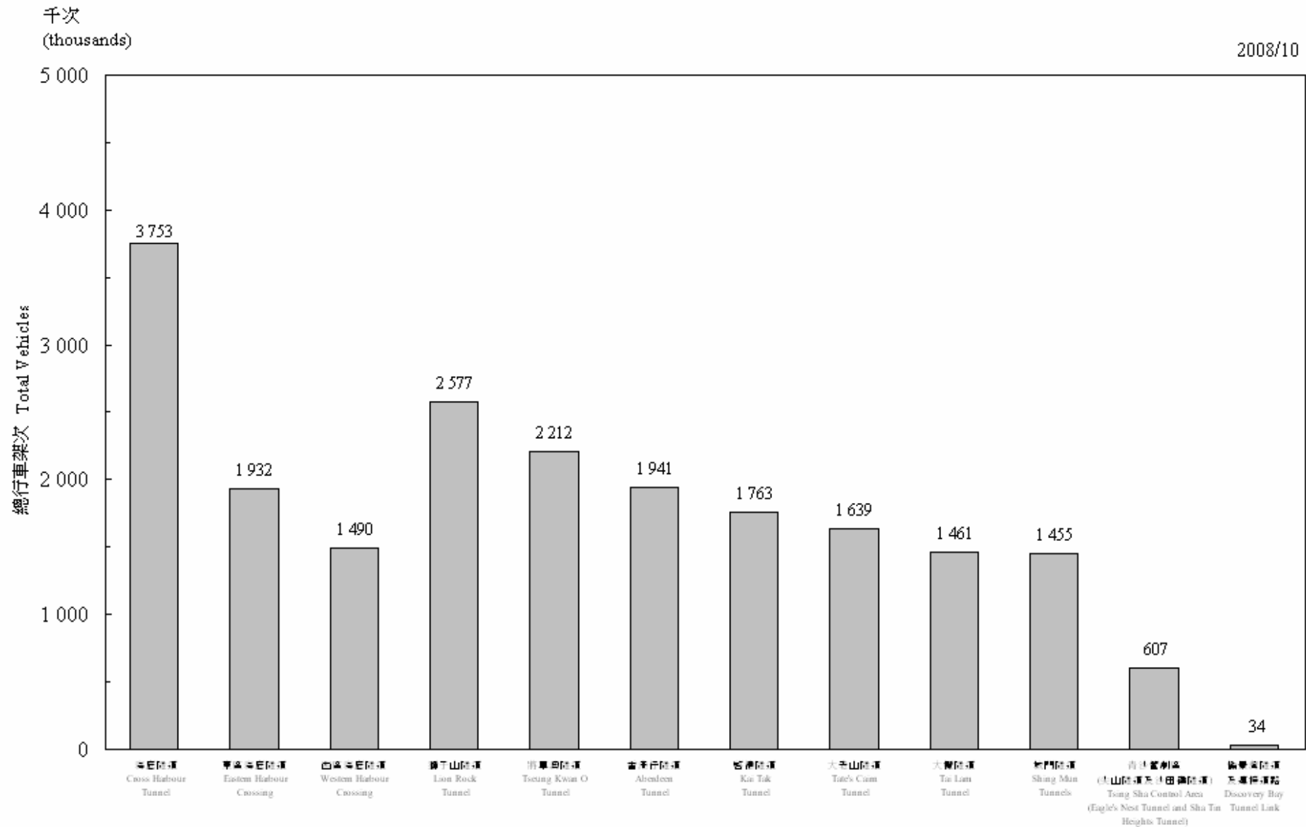
圖 3.1 - 隧道交通流量 (2008年10月) Chart 3.1 - Vehicular Traffic Through Tunnels (October 2008)
