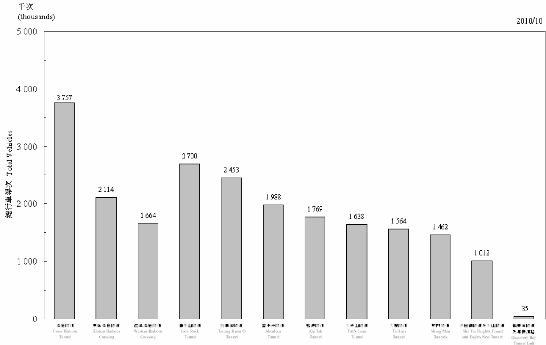
圖 3.1 - 隧道汽車流量 (2010年10月) Chart 3.1 - Vehicular Flow Through Tunnels (October 2010)
