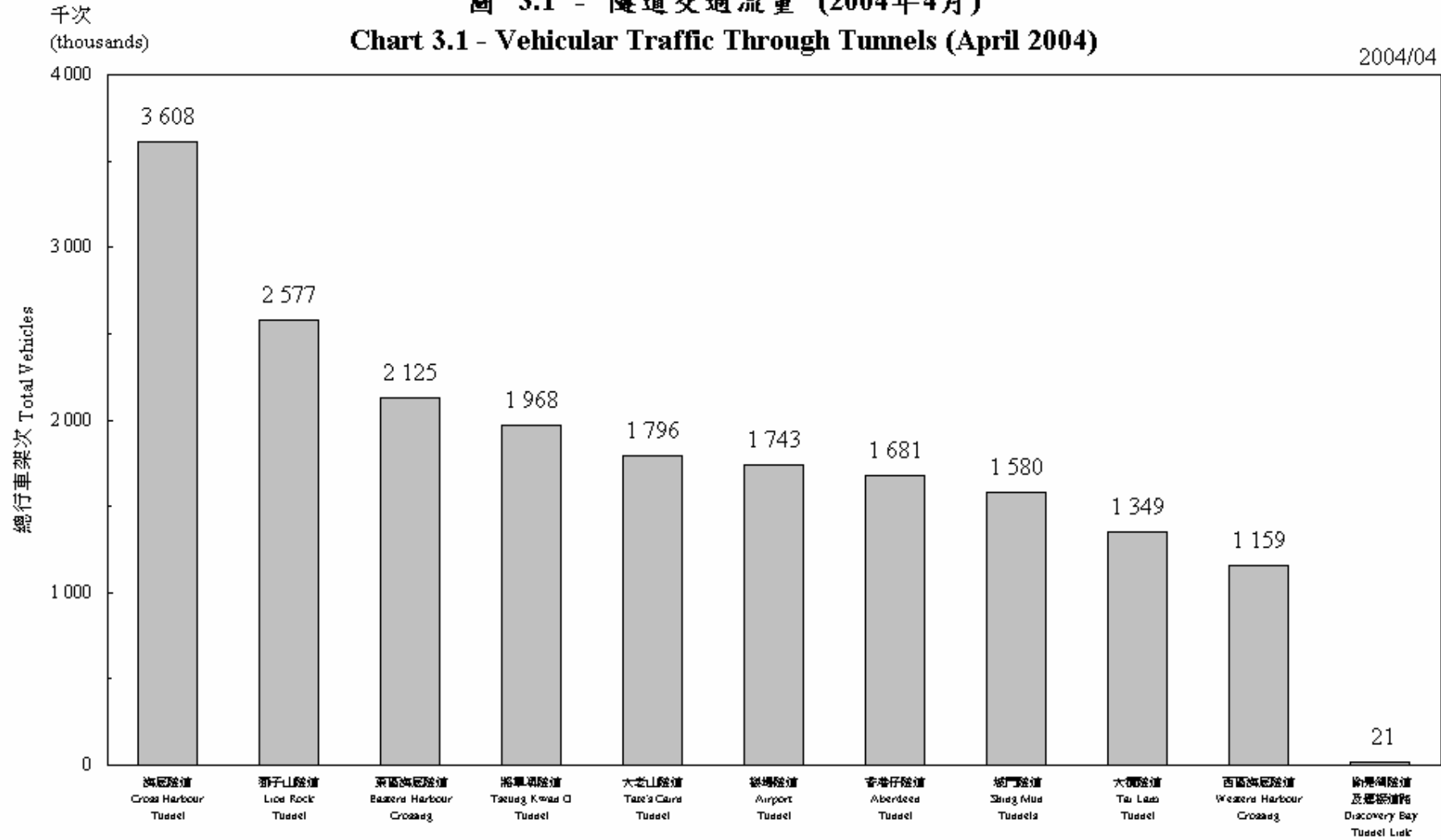
圖 3.1 - 隧道交通流量 (2004年4月)
