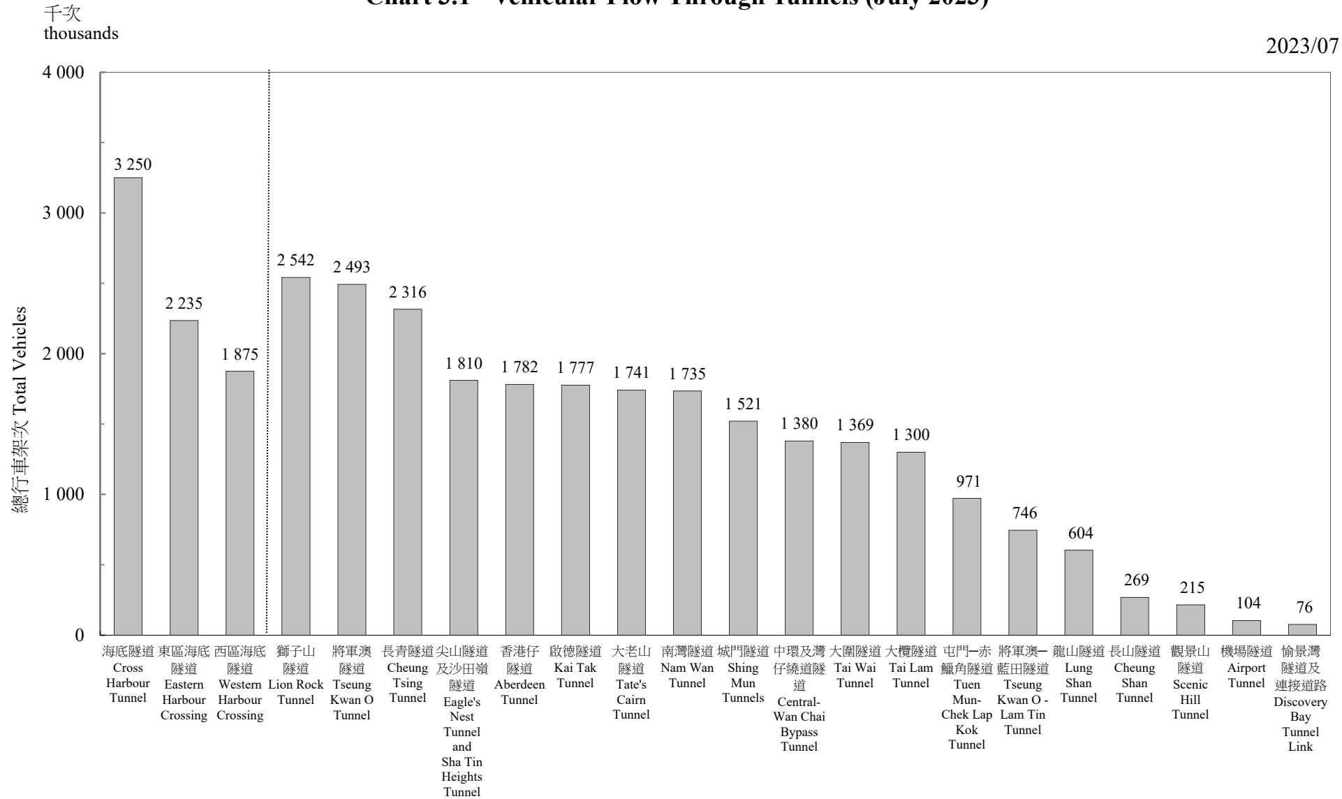
圖 3.1 - 隧道汽車流量 (二零二三年七月) Chart 3.1 - Vehicular Flow Through Tunnels (July 2023)
