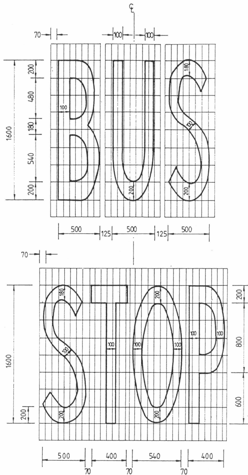
在豪華巴士及雙層巴士站使用的「BUS STOP」字母的尺寸
