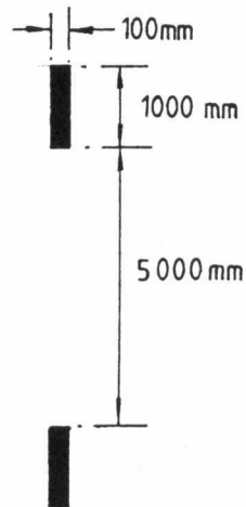
圖601 行車線劃線
