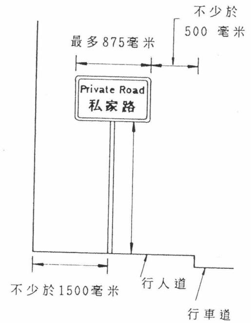
(iii) 用單柱支撐的標誌
