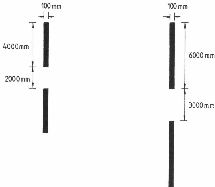
圖603 警告線
