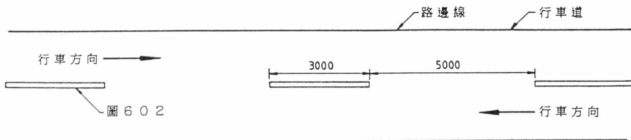
(i) 雙線雙程道路的車道中線標記
