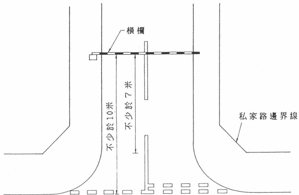
橫欄位置
