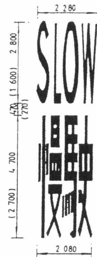
圖 6 1 5
