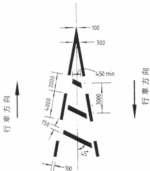
道路標記 1 1 2 7 號 斜線標記
