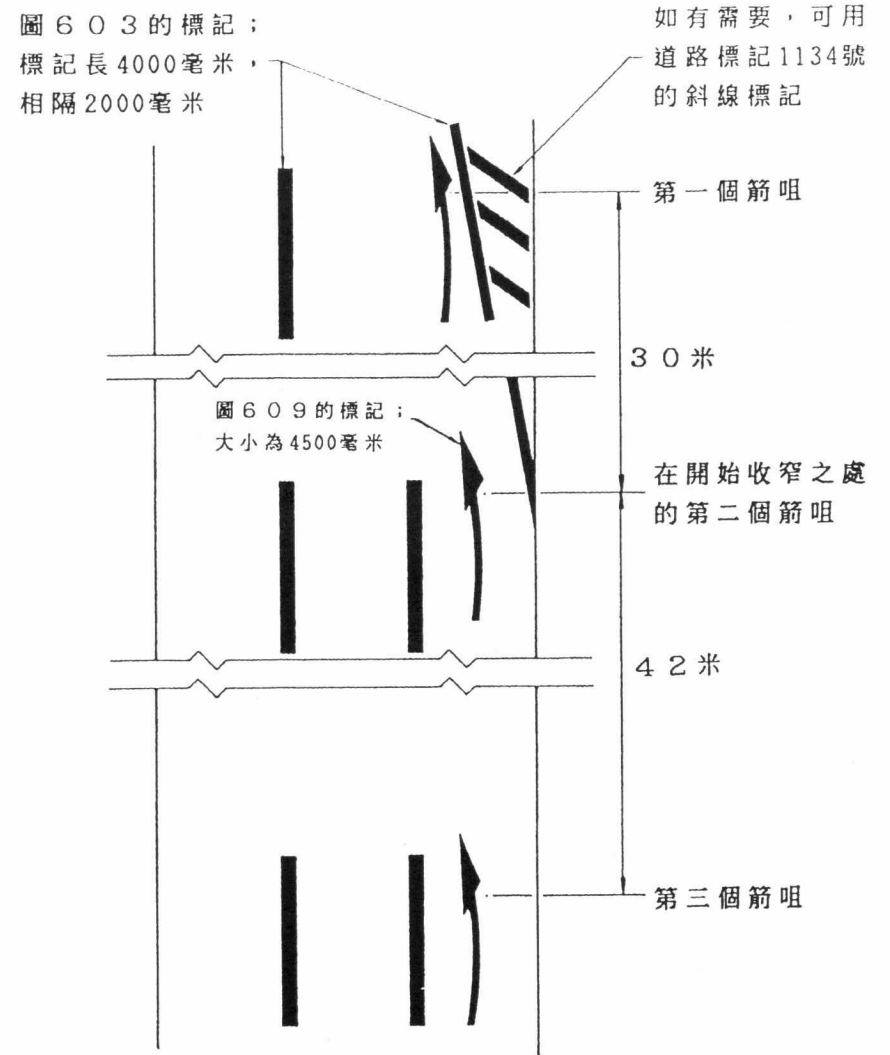
在單程路上使用圖 6 0 9 的警告箭咀
