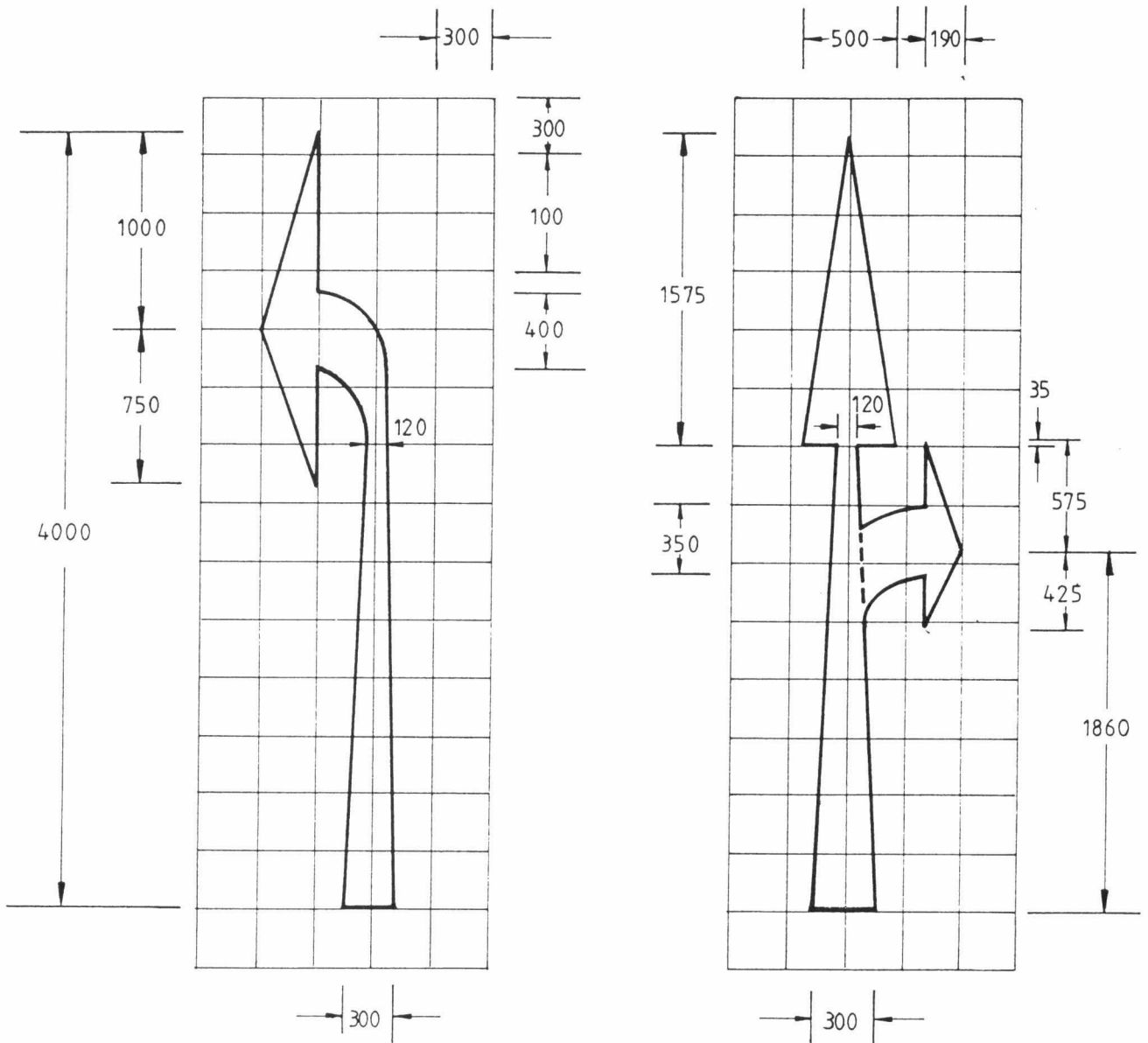
左轉箭咀 (方向相反則為右轉箭咀)
