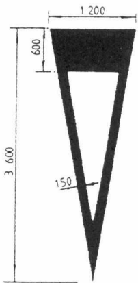
讓路符號 圖 6 0 8
