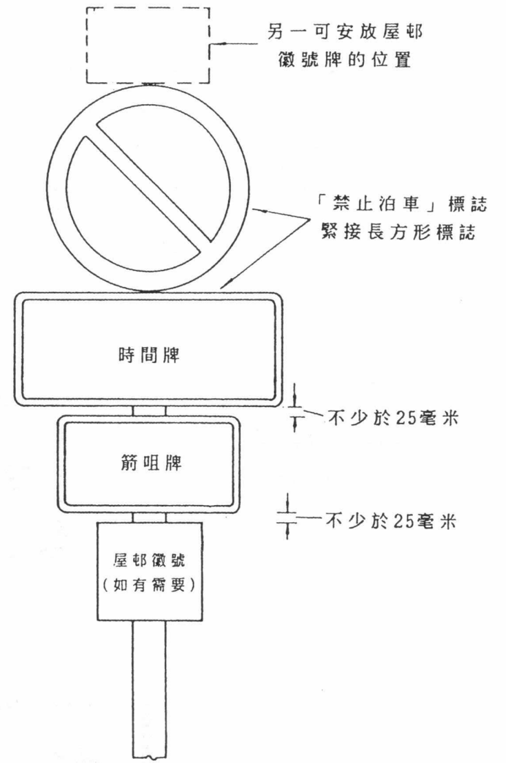
標誌牌組合
