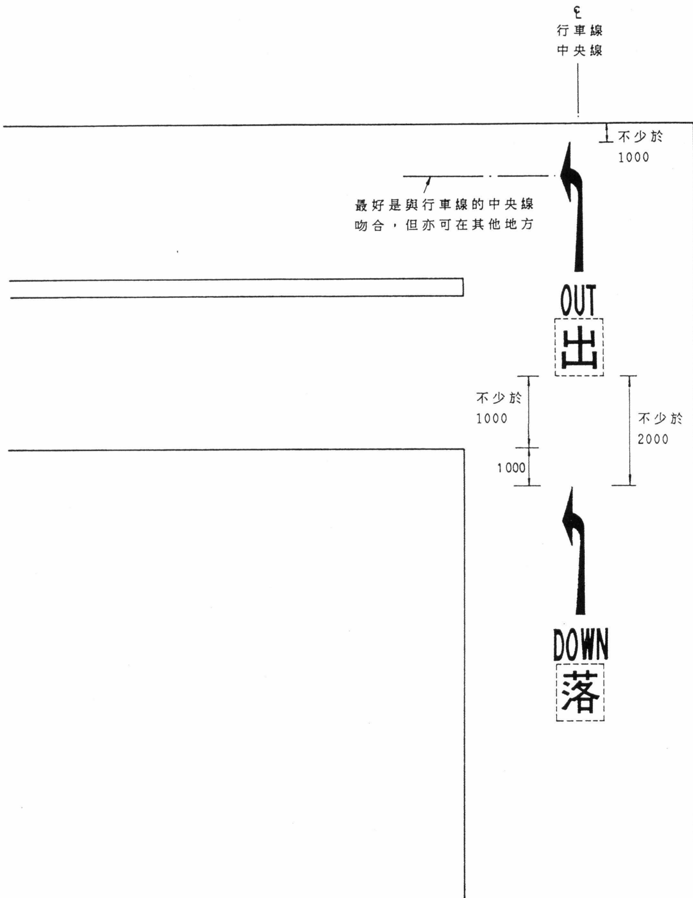
在相鄰的斜坡或類似地點設置標記
