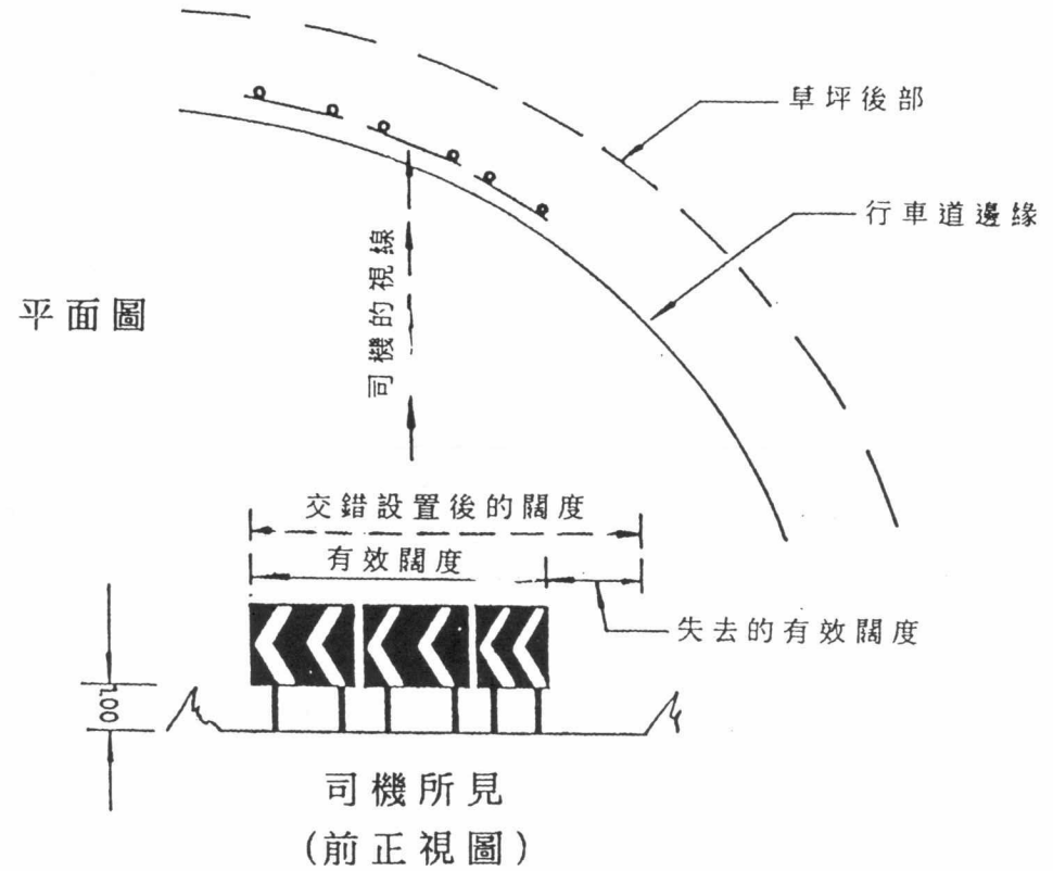
(ii) 不正確排列
