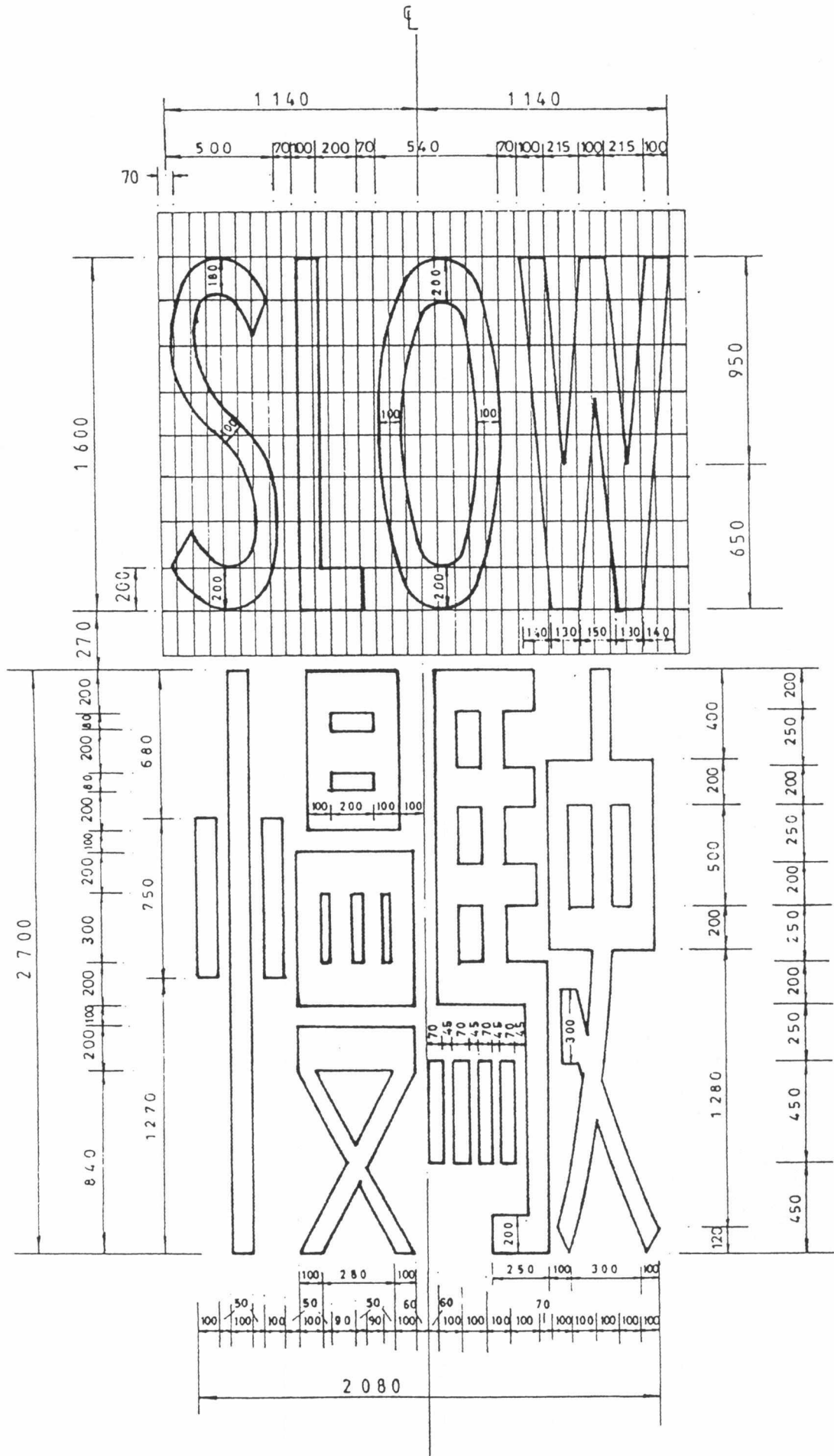
圖 6 0 5 的 結 構 詳 情
