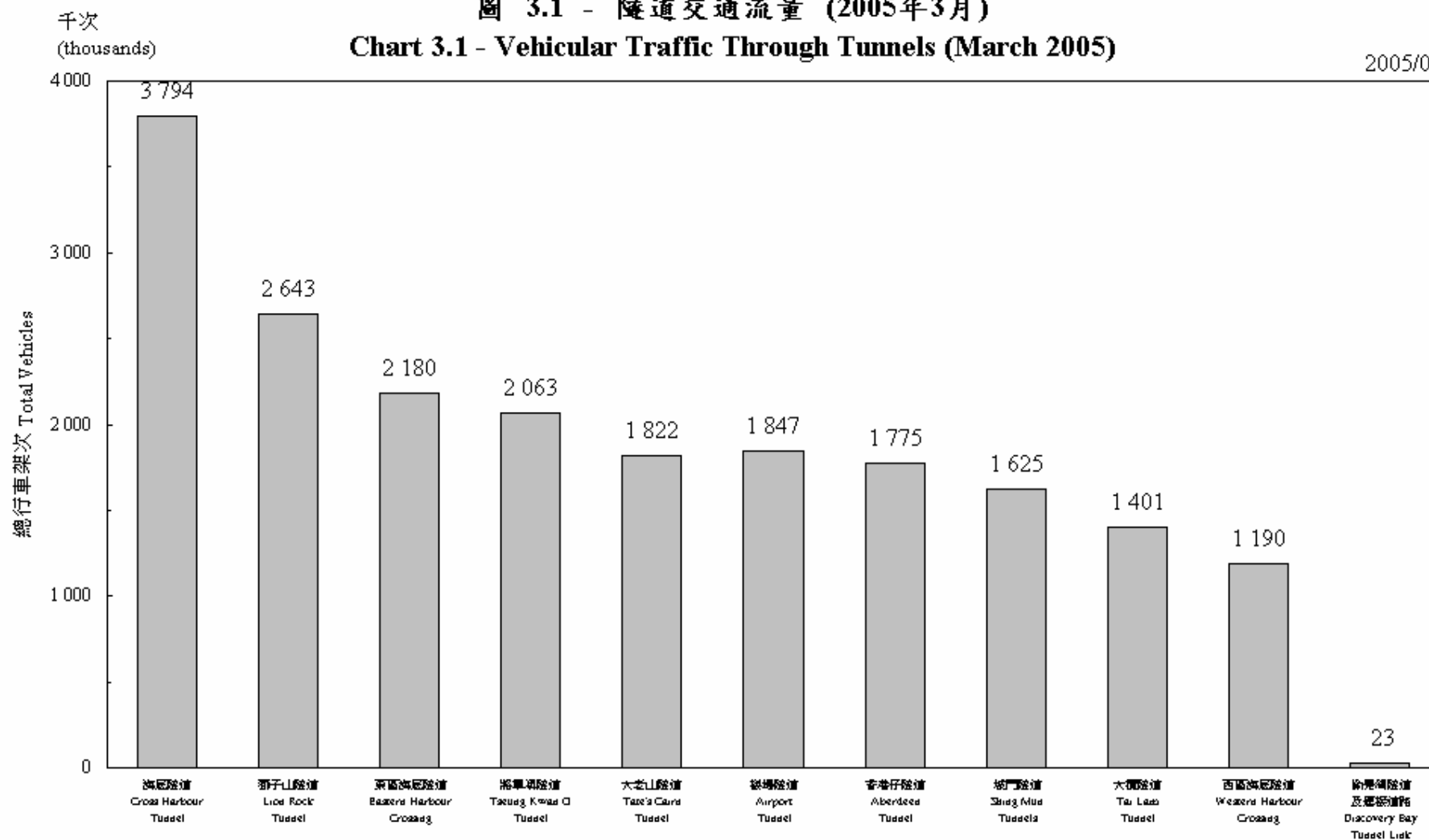
圖 3.1 - 隧道交通流量 (2005年3月)
