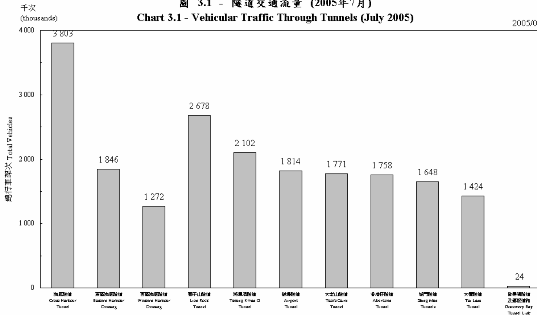
圖 3.1 - 隧道交通流量 (2005年7月)
