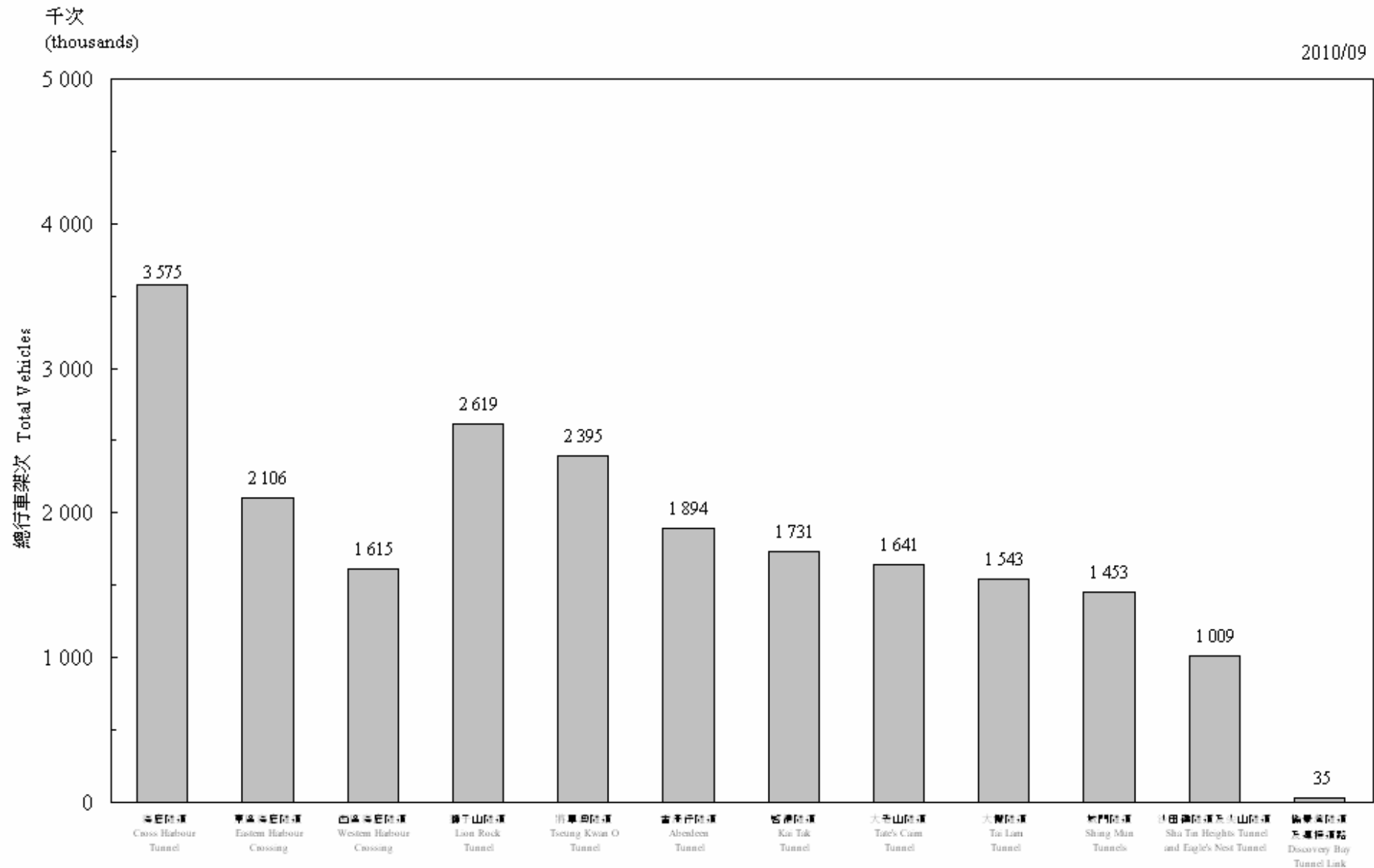
圖 3.1 - 隧道汽車流量 (2010年9月) Chart 3.1 - Vehicular Flow Through Tunnels (September 2010)
