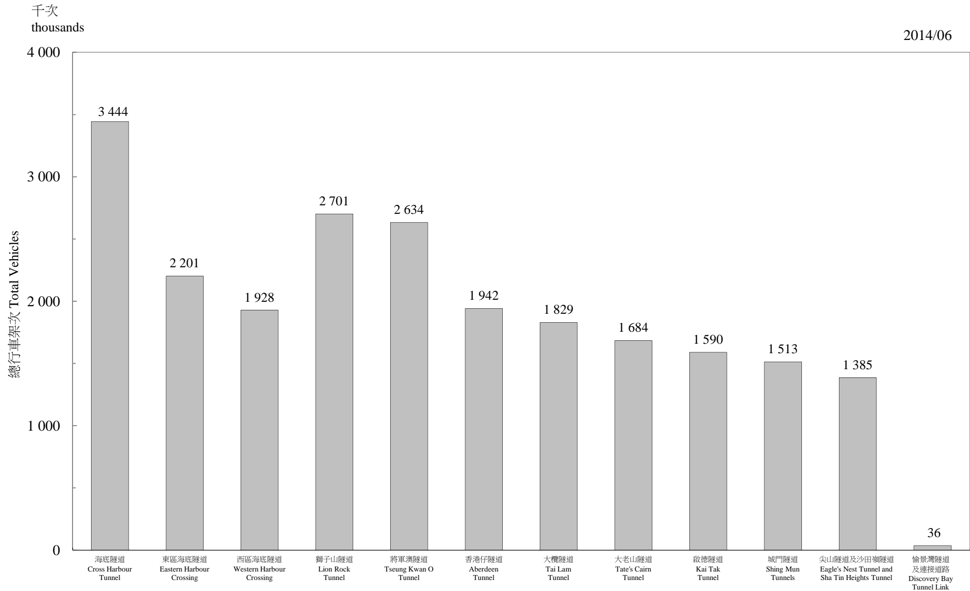
圖 3.1 - 隧道汽車流量 (二零一四年六月) Chart 3.1 - Vehicular Flow Through Tunnels (June 2014)
