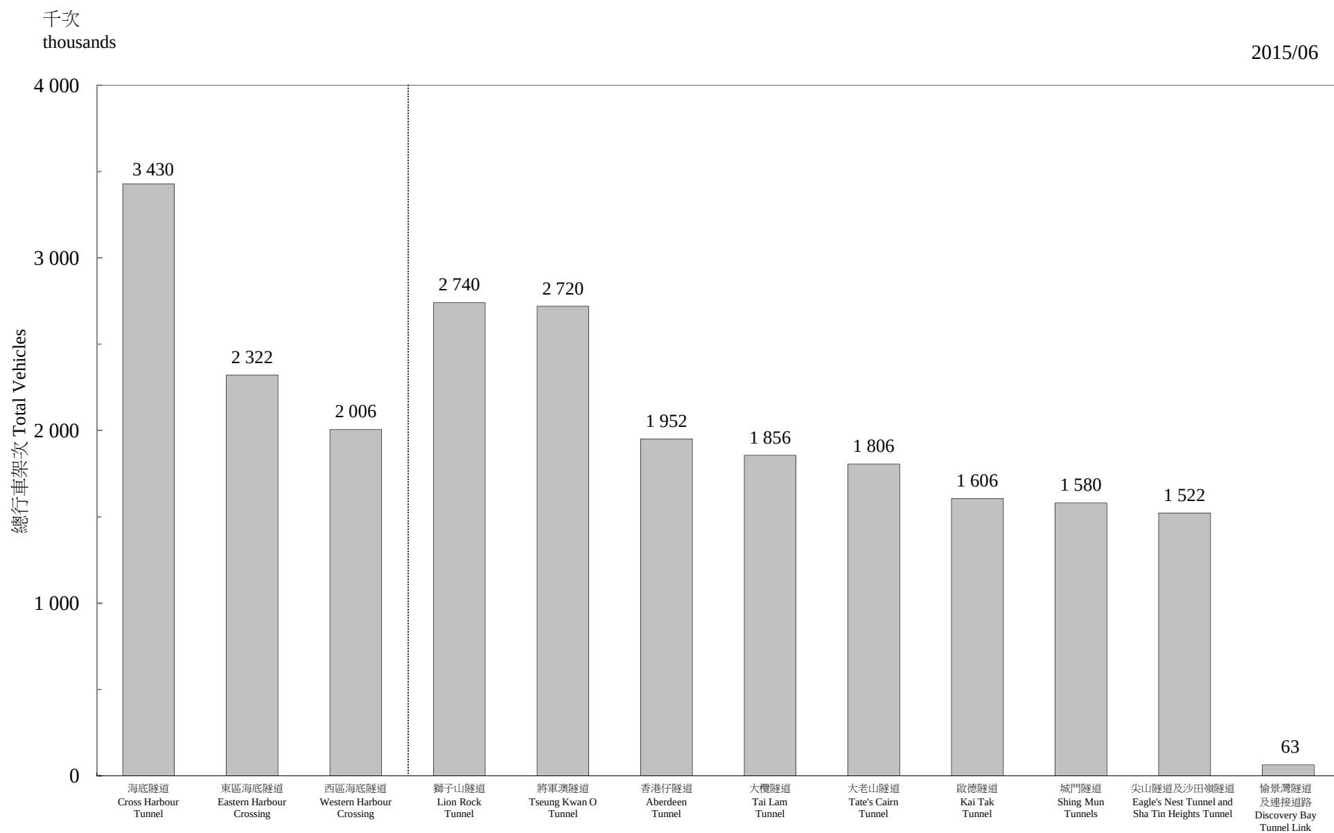
圖 3.1 - 隧道汽車流量 (二零一五年六月) Chart 3.1 - Vehicular Flow Through Tunnels (June 2015)
