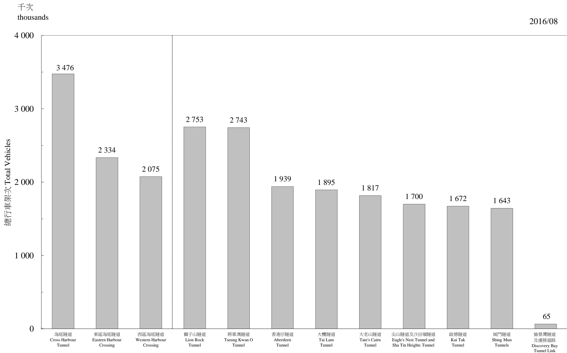
圖 3.1 - 隧道汽車流量 (二零一六年八月) Chart 3.1 - Vehicular Flow Through Tunnels (August 2016)
