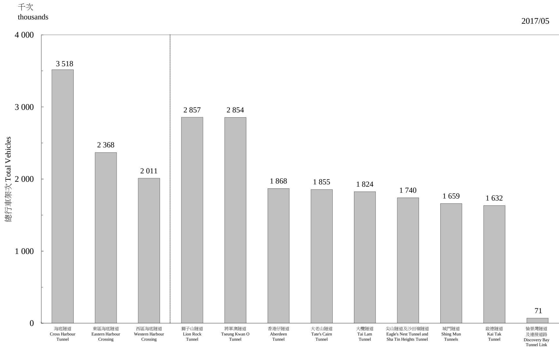
圖 3.1 - 隧道汽車流量 (二零一七年五月) Chart 3.1 - Vehicular Flow Through Tunnels (May 2017)
