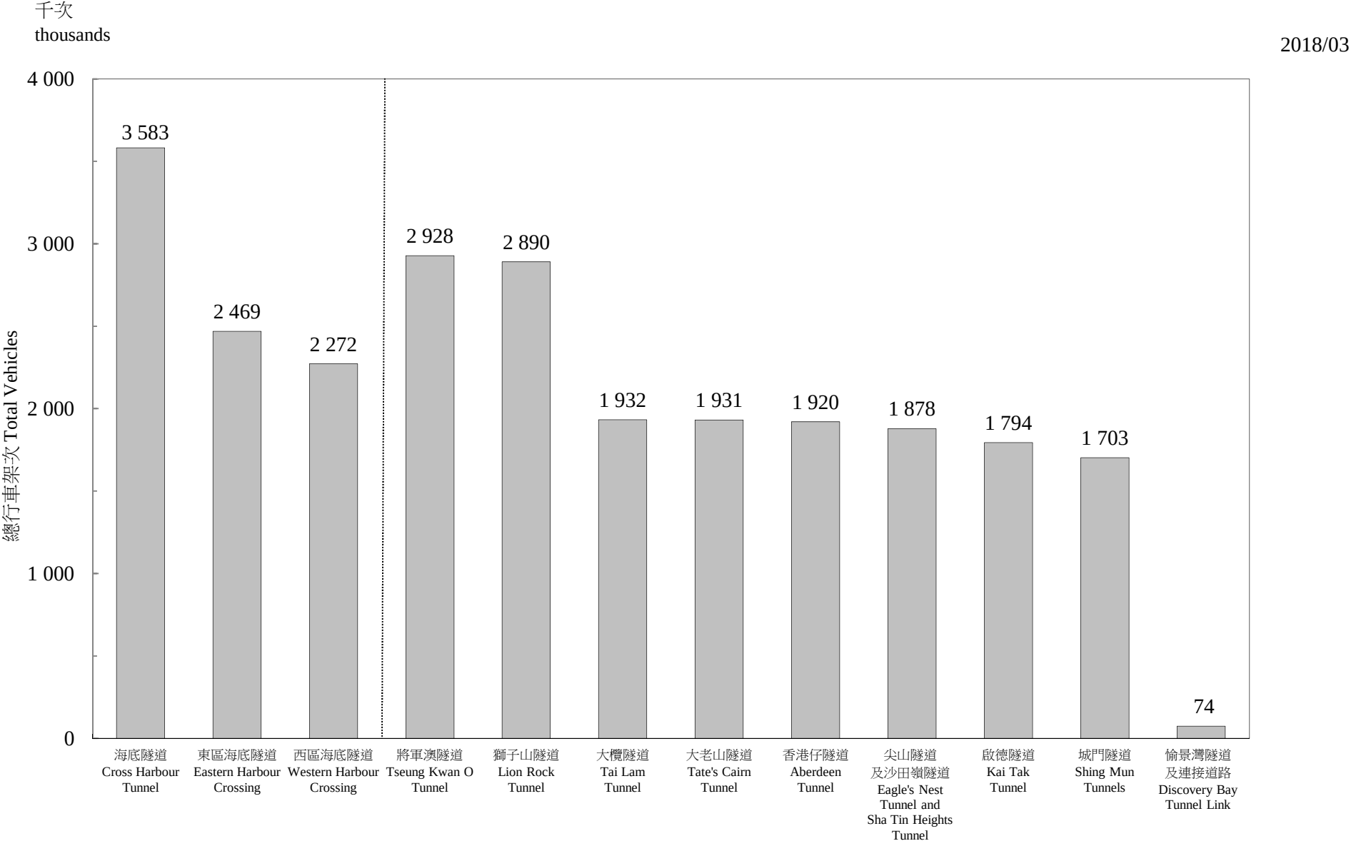
圖 3.1 - 隧道汽車流量 (二零一八年三月) Chart 3.1 - Vehicular Flow Through Tunnels (March 2018)
