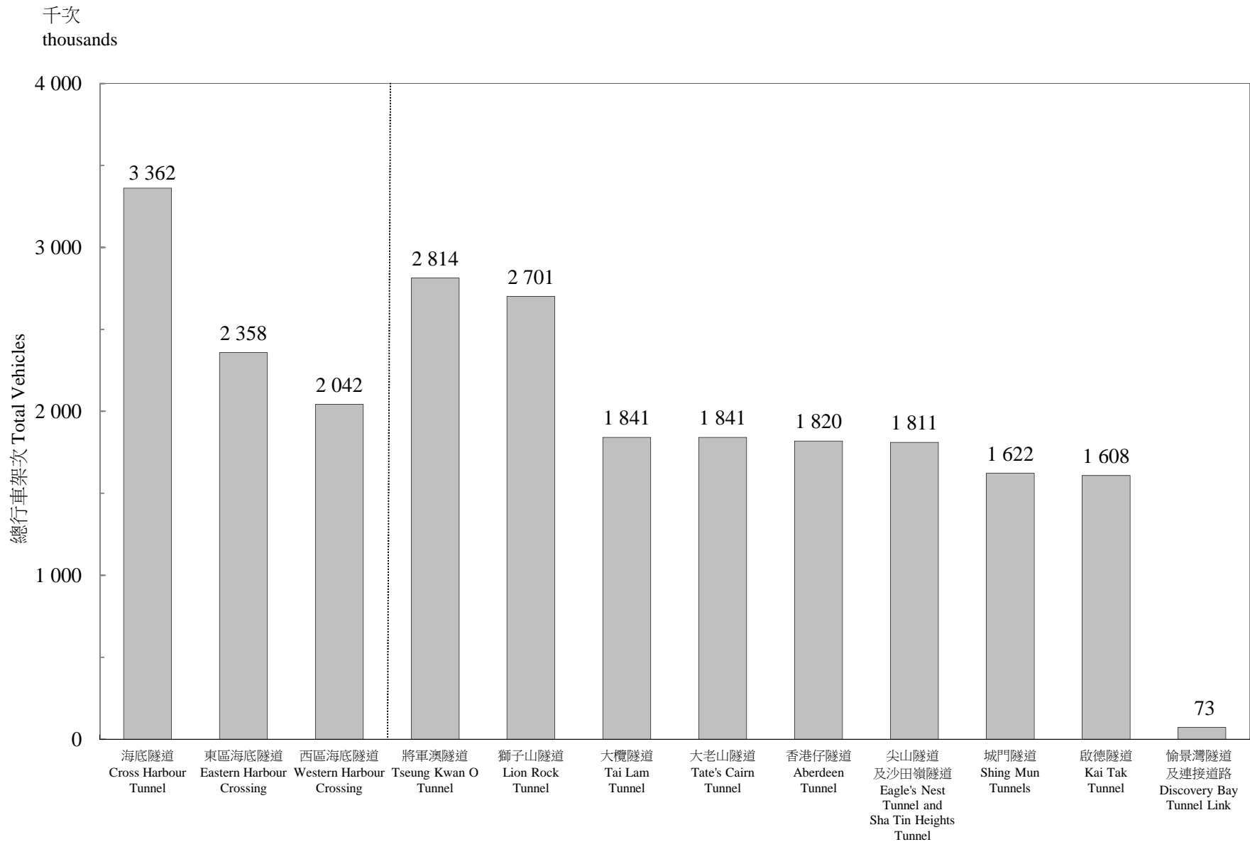
圖 3.1 - 隧道汽車流量 (二零一八年六月) Chart 3.1 - Vehicular Flow Through Tunnels (June 2018)
