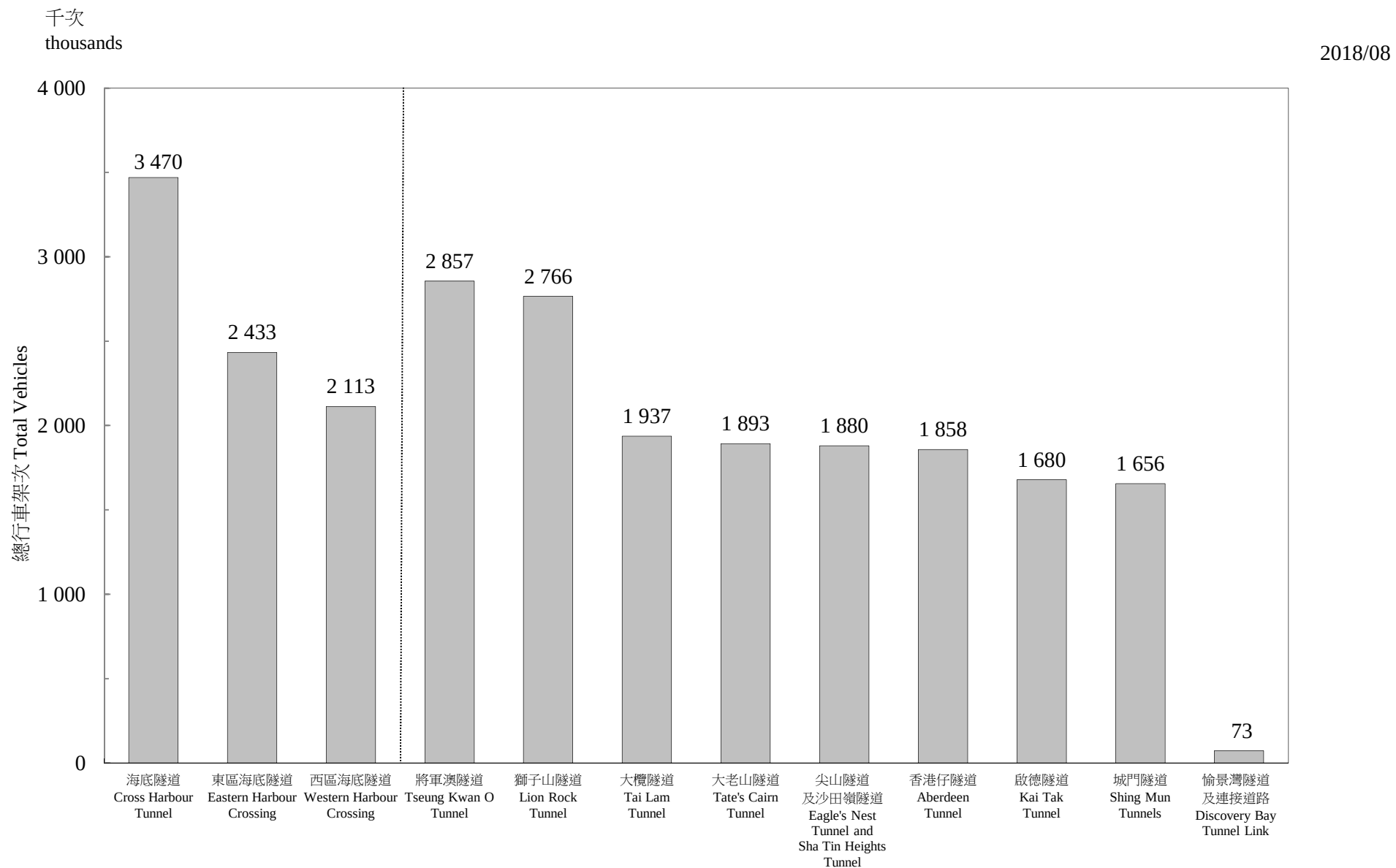
圖 3.1 - 隧道汽車流量 (二零一八年八月) Chart 3.1 - Vehicular Flow Through Tunnels (August 2018)
