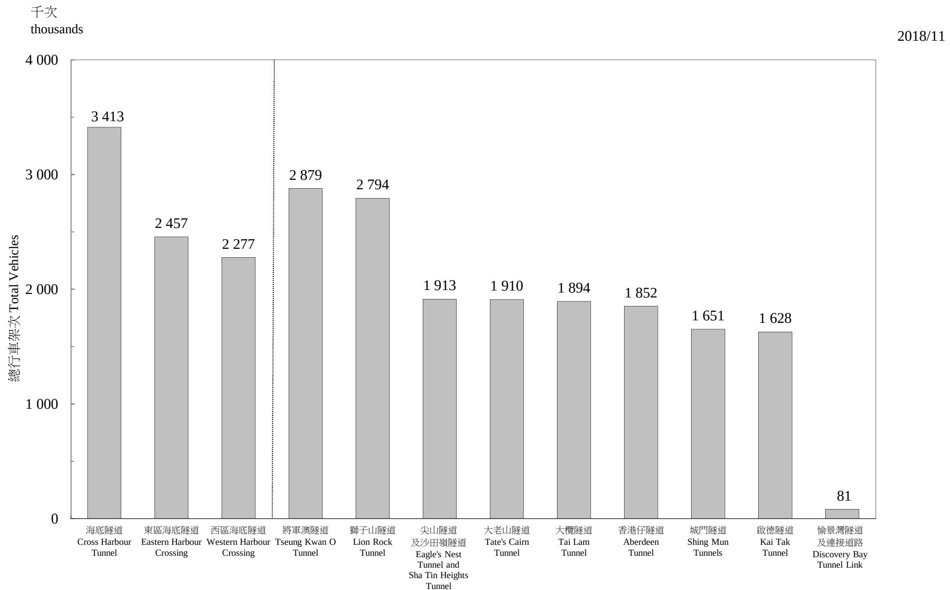
圖 3.1 - 隧道汽車流量 (二零一八年十一月) Chart 3.1 - Vehicular Flow Through Tunnels (November 2018)
