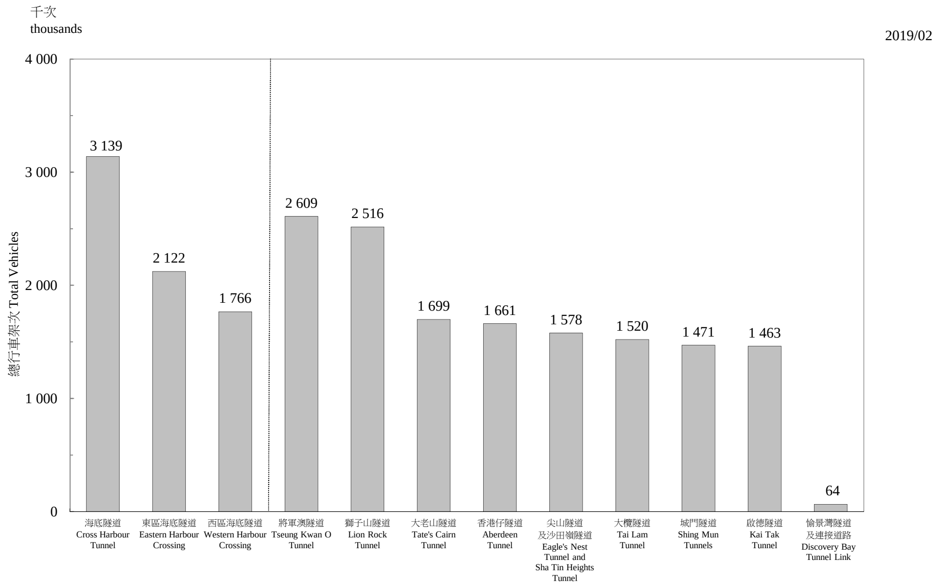
圖 3.1 - 隧道汽車流量 (二零一九年二月) Chart 3.1 - Vehicular Flow Through Tunnels (February 2019)
