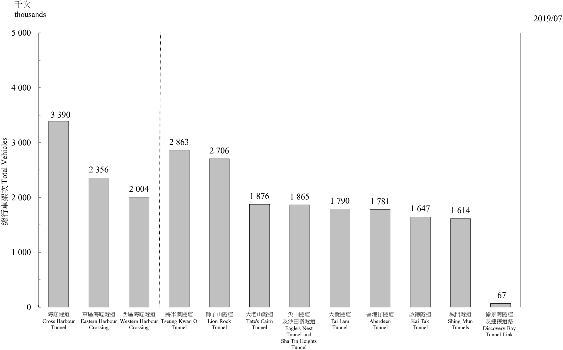
圖 3.1 - 隧道汽車流量 (二零一九年七月) Chart 3.1 - Vehicular Flow Through Tunnels (July 2019)
