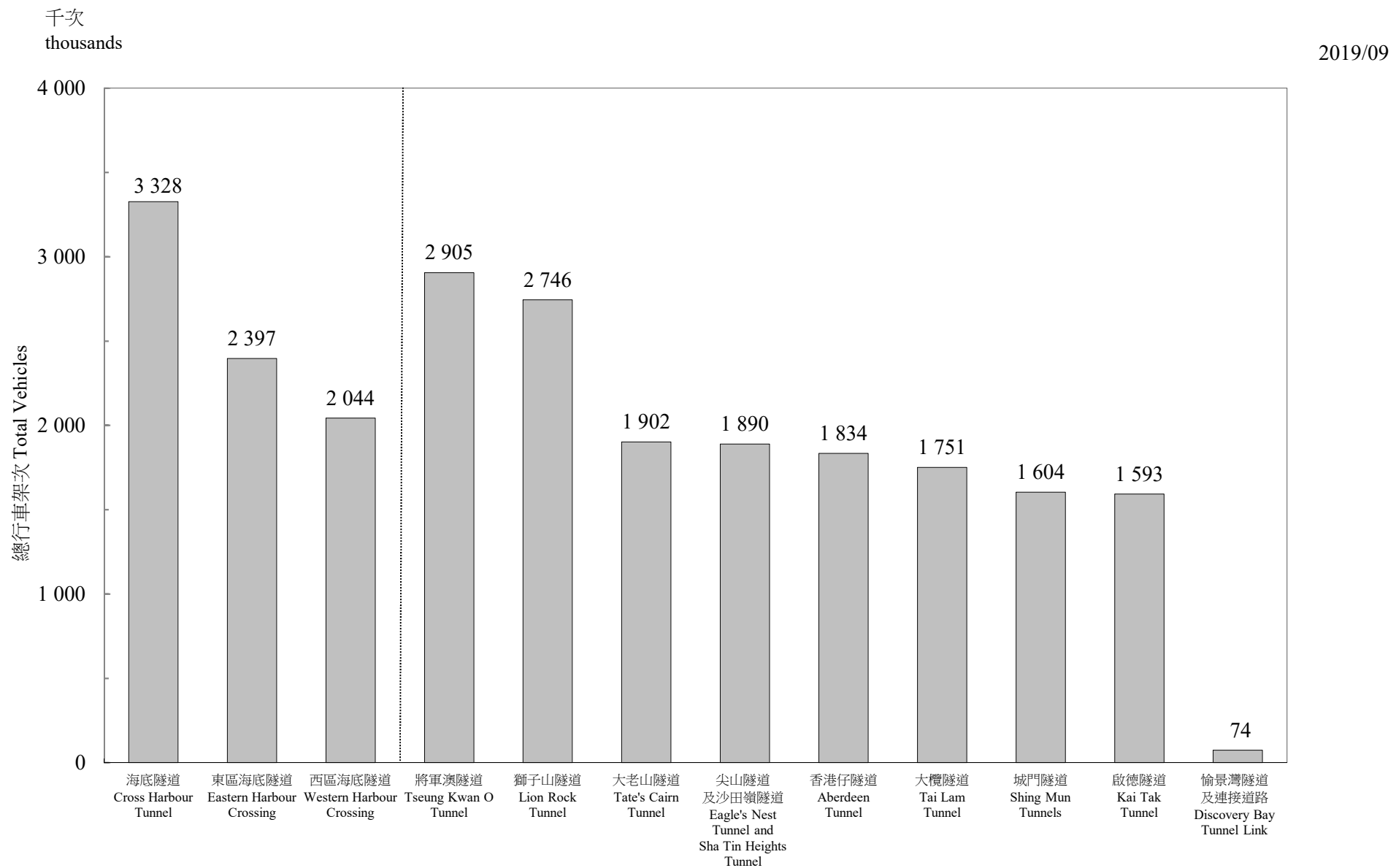
圖 3.1 - 隧道汽車流量 (二零一九年九月) Chart 3.1 - Vehicular Flow Through Tunnels (September 2019)
