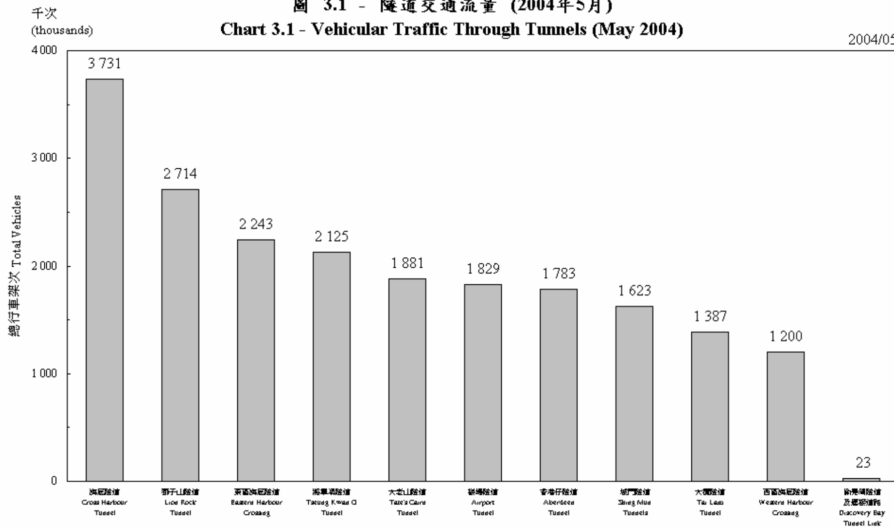
圖 3.1 - 隧道交通流量 (2004年5月)
