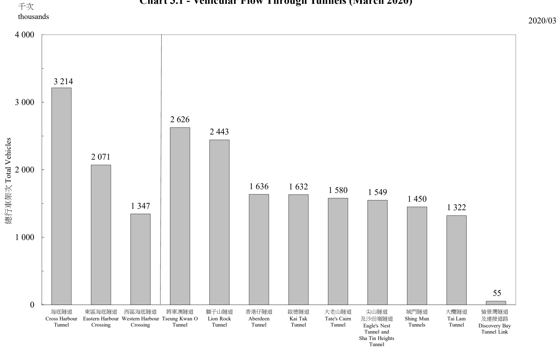
圖 3.1 - 隧道汽車流量 (二零二零年三月) Chart 3.1 - Vehicular Flow Through Tunnels (March 2020)
