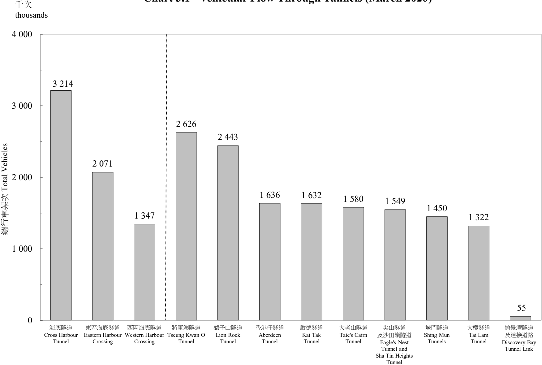
圖 3.1 - 隧道汽車流量 (二零二零年三月) Chart 3.1 - Vehicular Flow Through Tunnels (March 2020)
