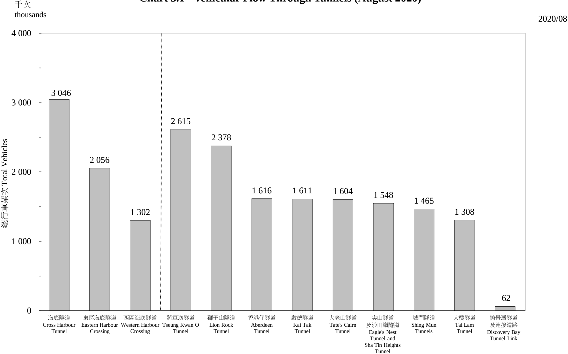
圖 3.1 - 隧道汽車流量 (二零二零年八月) Chart 3.1 - Vehicular Flow Through Tunnels (August 2020)
