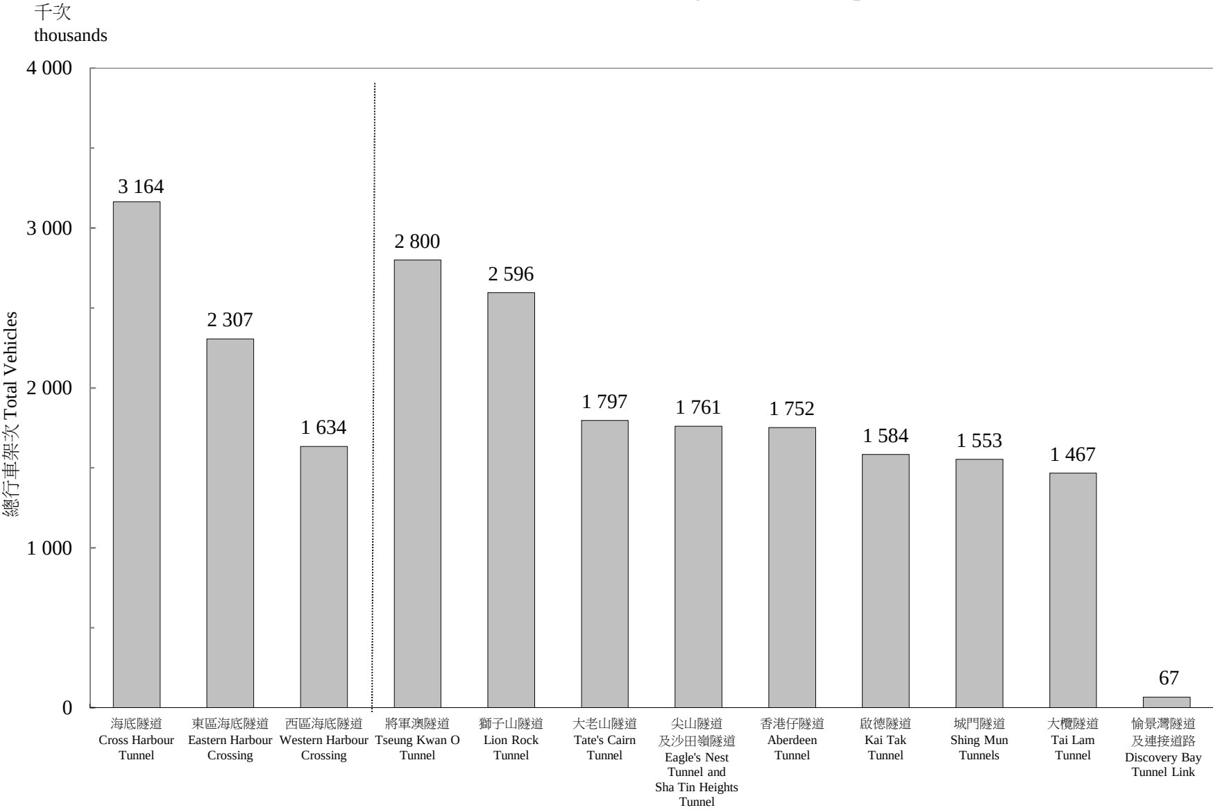
圖 3.1 - 隧道汽車流量 (二零二零年九月) Chart 3.1 - Vehicular Flow Through Tunnels (September 2020)
