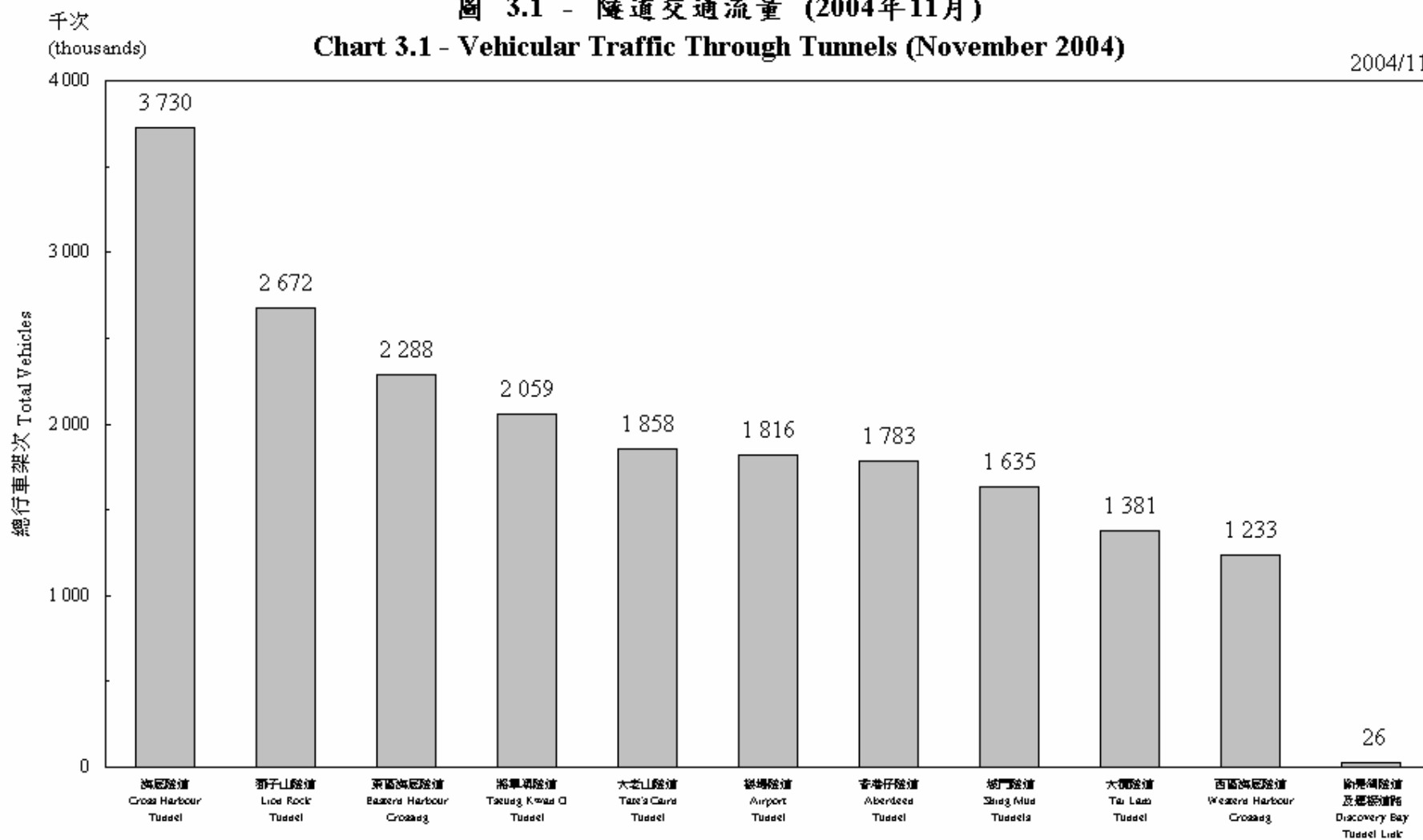
圖 3.1 - 隧道交通流量 (2004年11月)
