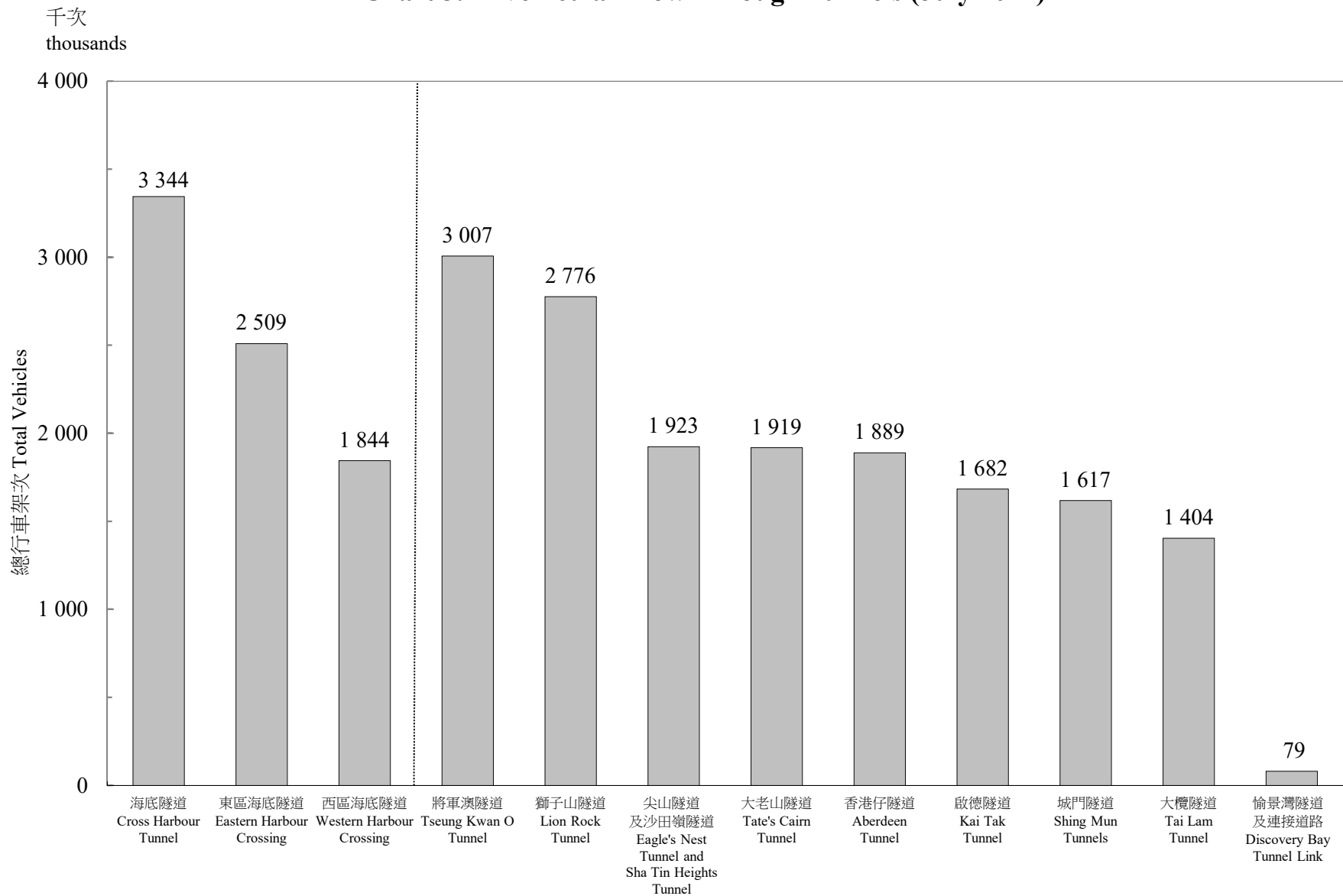
圖 3.1 - 隧道汽車流量 (二零二一年七月) Chart 3.1 - Vehicular Flow Through Tunnels (July 2021)
