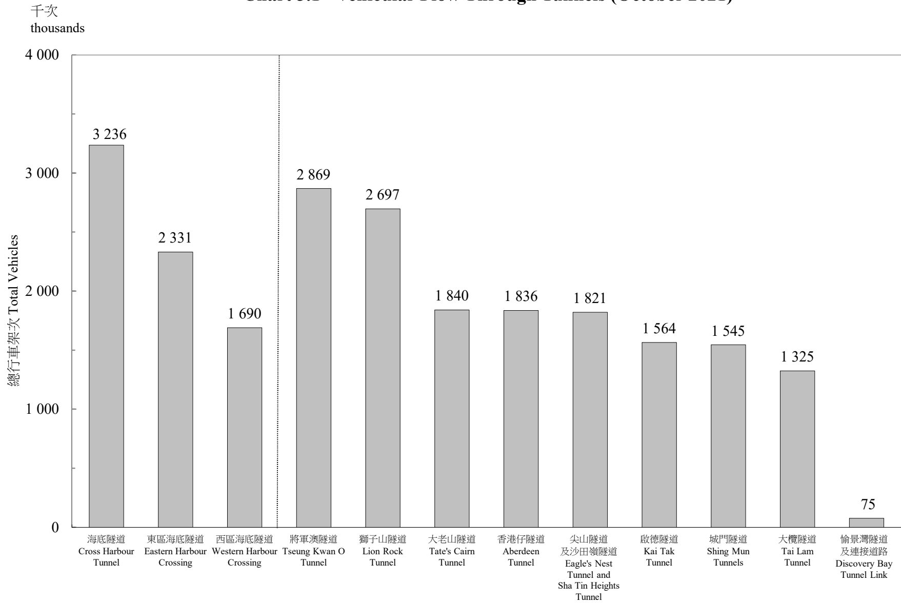
圖 3.1 - 隧道汽車流量 (二零二一年十月) Chart 3.1 - Vehicular Flow Through Tunnels (October 2021)
