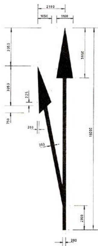
RM 1125
