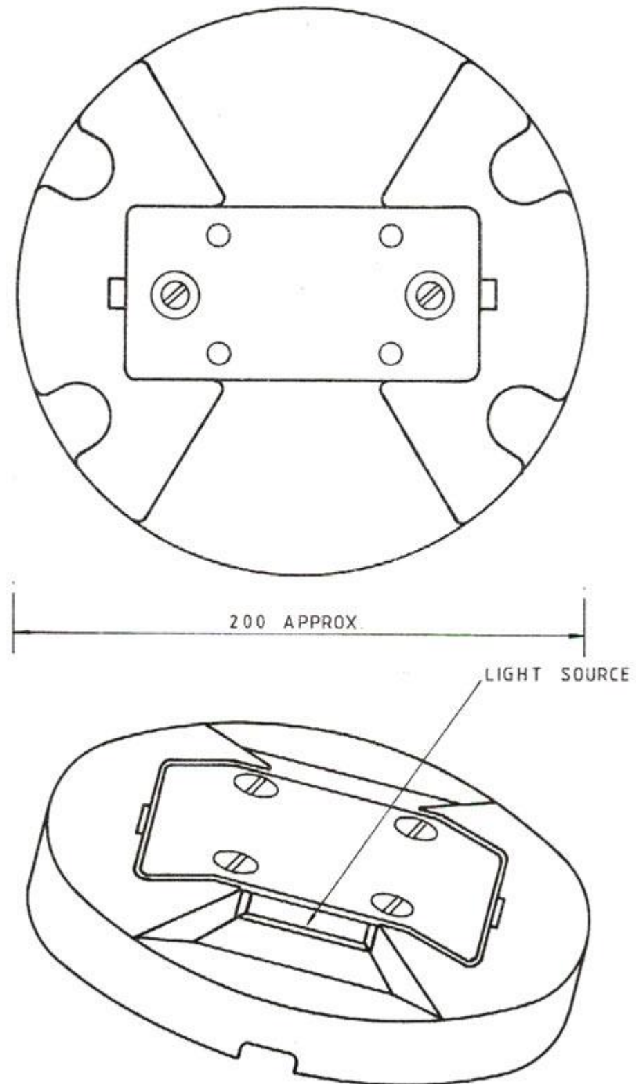
DIAGRAM 5.5.2.4 : PAVEMENT LIGHTS
