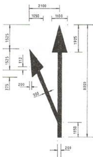
RM 1125
