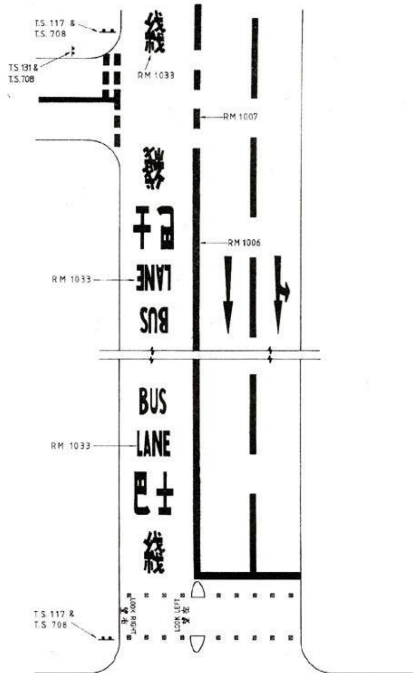
DIAGRAM 5.9.3.1 : CONTRA FLOW BUS LANE
