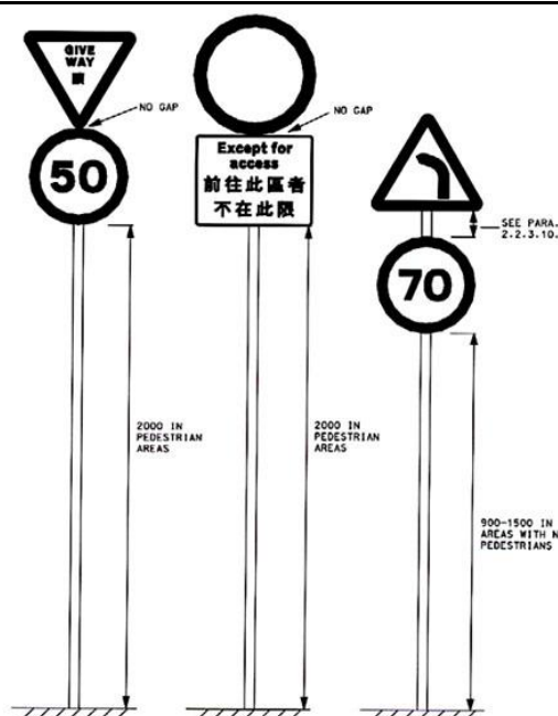
DIAGRAM 2.2.3.2 : SIGN ASSEMBLIES
