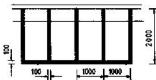
RM 1051 (PA 13)
