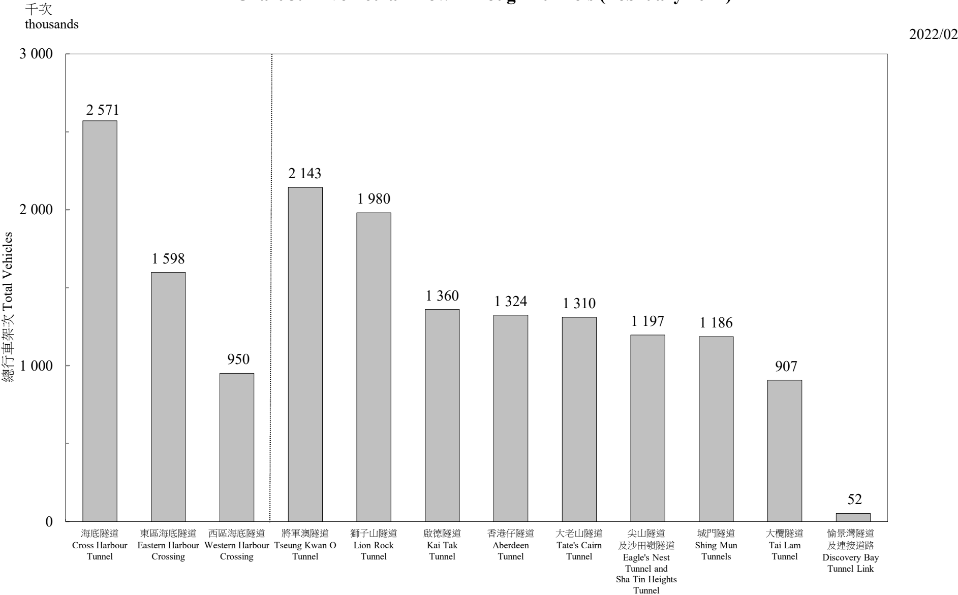
圖 3.1 - 隧道汽車流量 (二零二二年二月) Chart 3.1 - Vehicular Flow Through Tunnels (February 2022)
