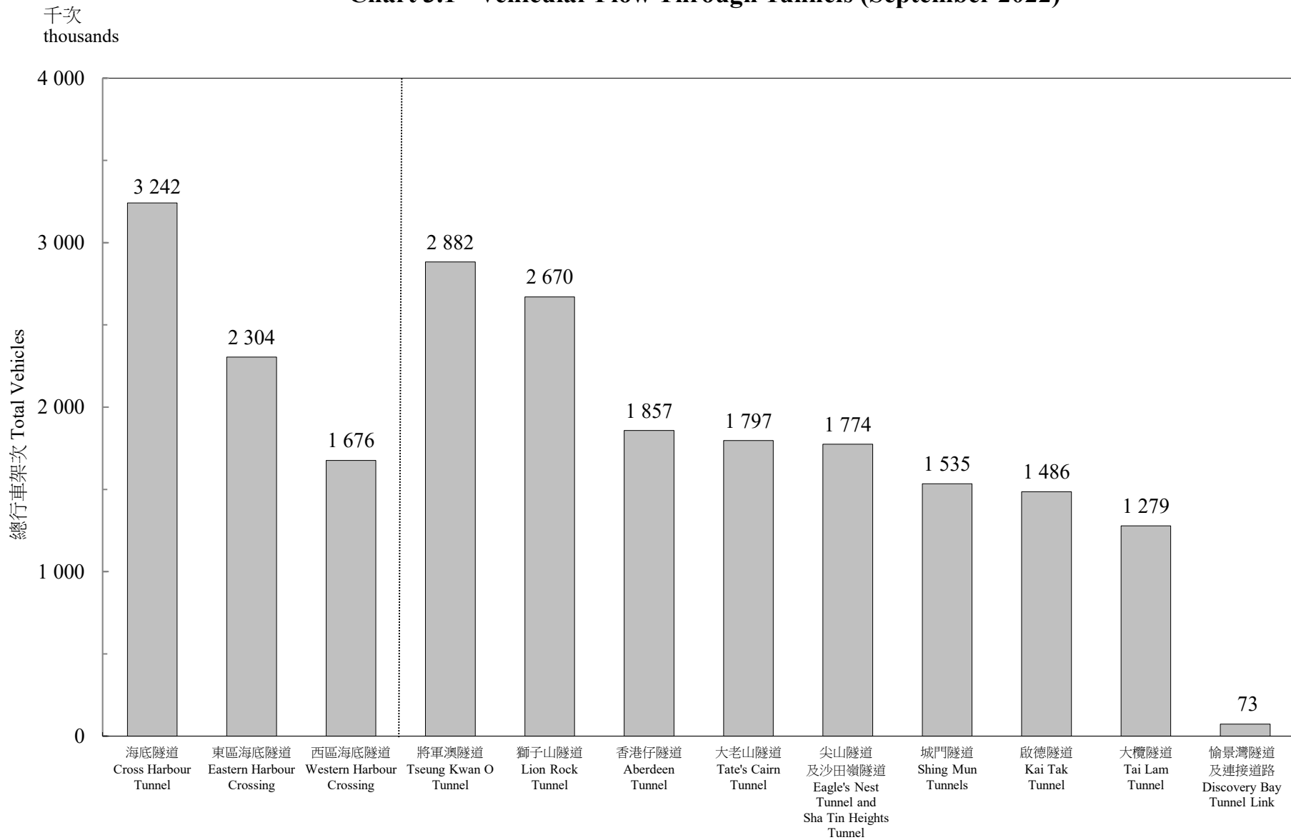
圖 3.1 - 隧道汽車流量 (二零二二年九月) Chart 3.1 - Vehicular Flow Through Tunnels (September 2022)
