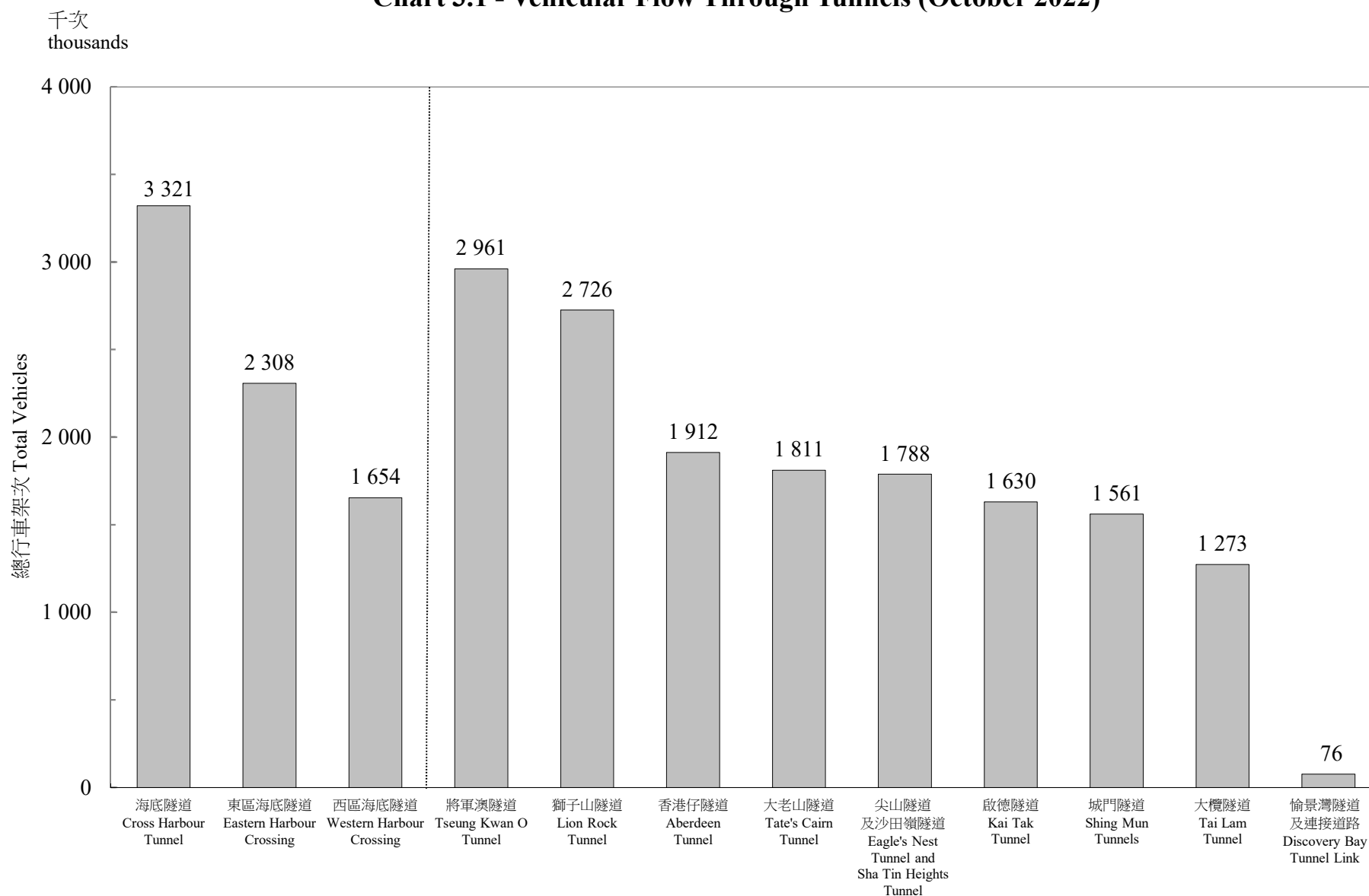
圖 3.1 - 隧道汽車流量 (二零二二年十月) Chart 3.1 - Vehicular Flow Through Tunnels (October 2022)
