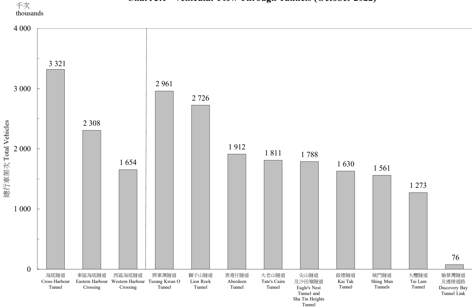
圖 3.1 - 隧道汽車流量 (二零二二年十月) Chart 3.1 - Vehicular Flow Through Tunnels (October 2022)
