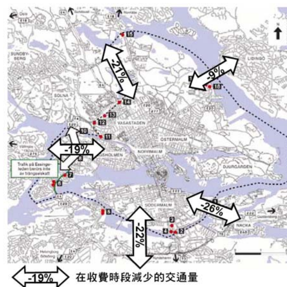
圖 3.10 斯德哥爾摩的擠塞收費試驗計劃－交通量減少
