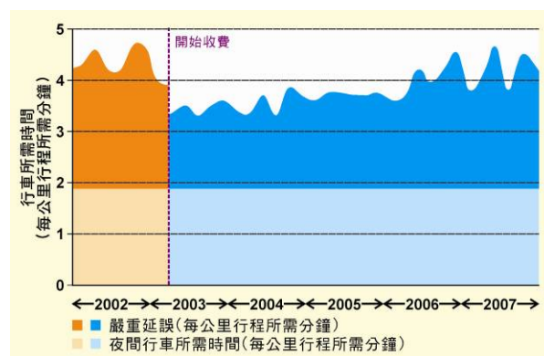
圖 3.9 倫敦區域擠塞收費計劃：實施前／後的行車所需時間和延誤程度
