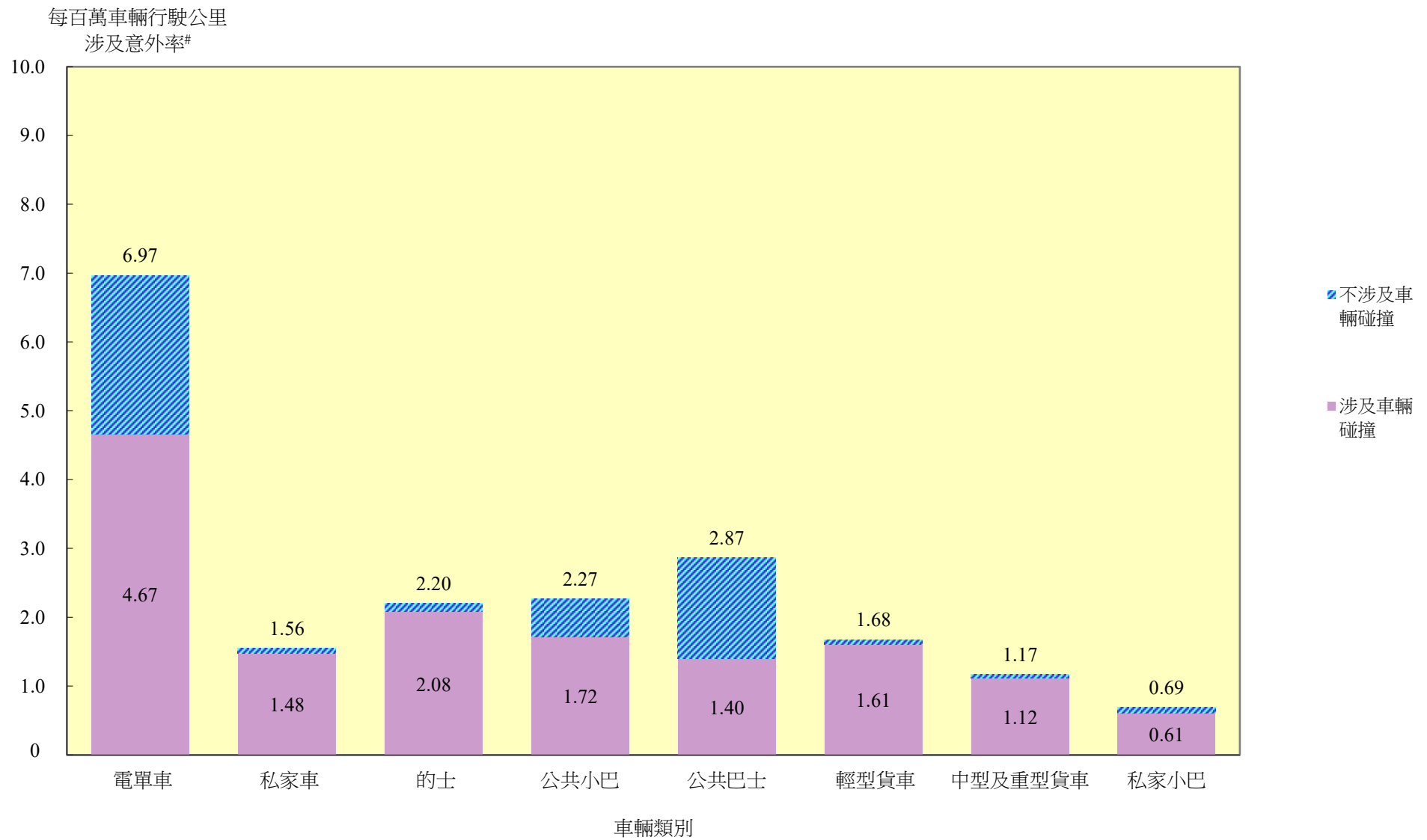
圖B11 - 二零二五年按選定車輛類別劃分的涉及意外率^
